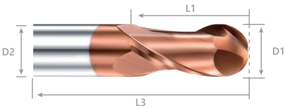
超微粒圓頭立銑刀 End Mills
