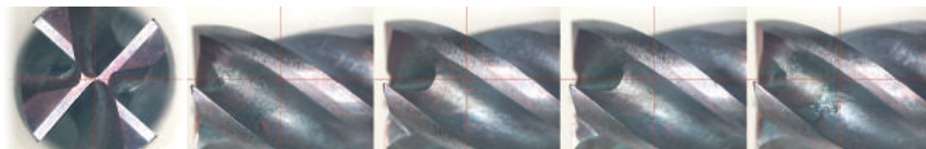
插銑圖型範例 Plunge Milling Example
